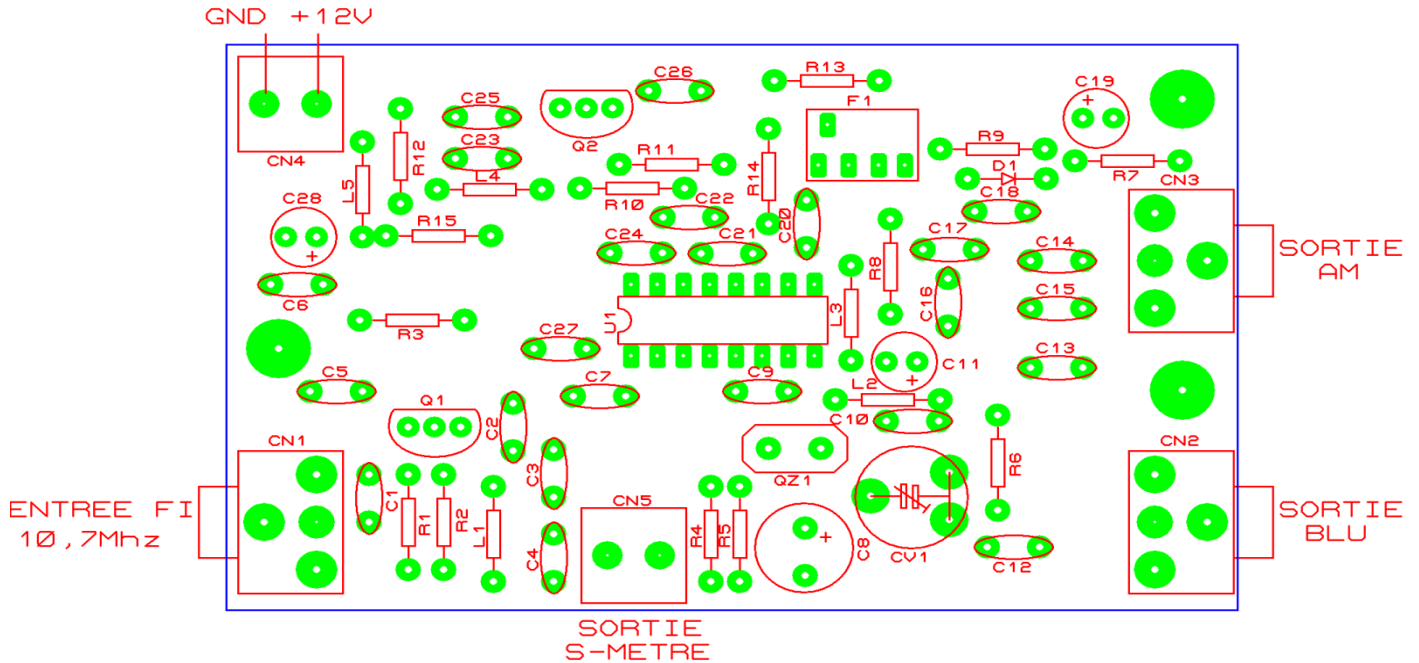
Schéma d'implantation
