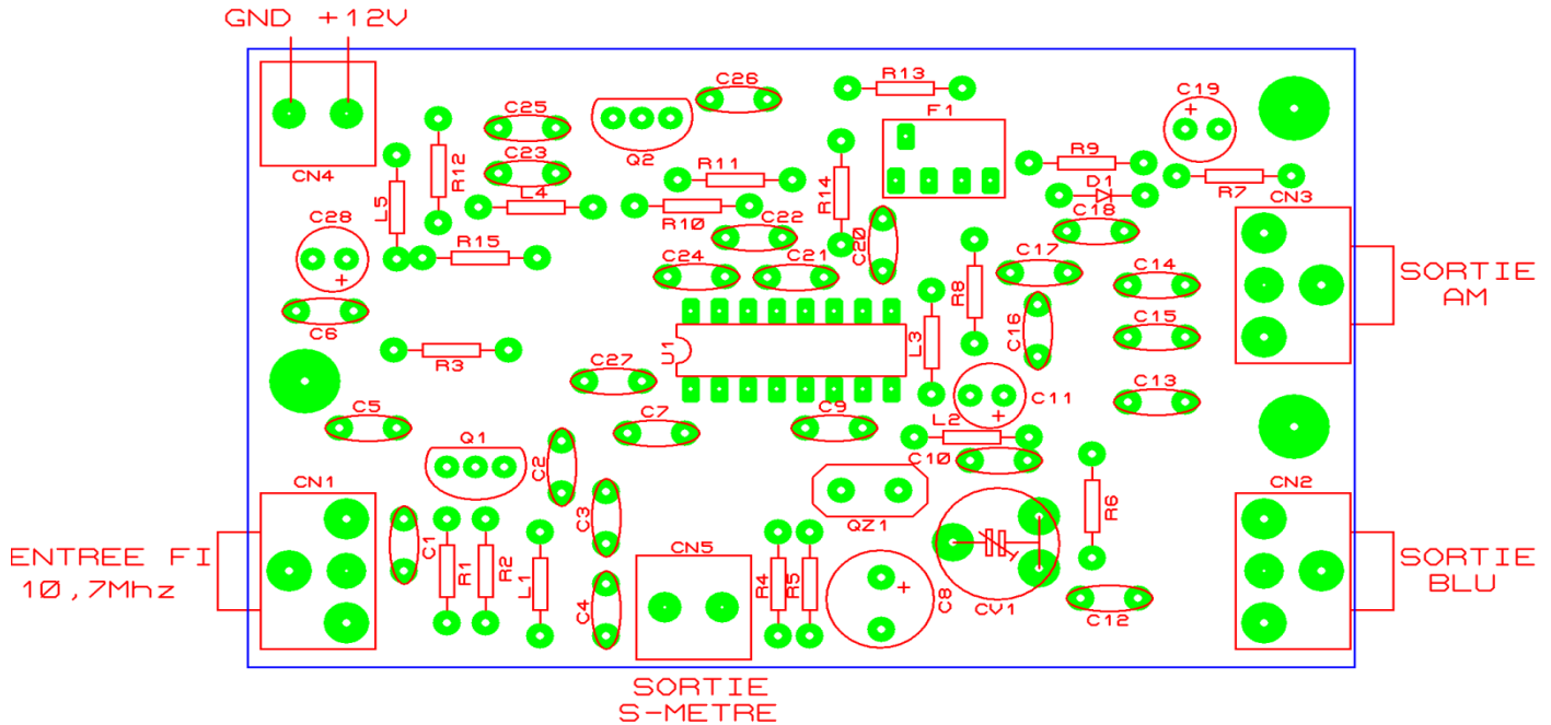
Schéma d'implantation
