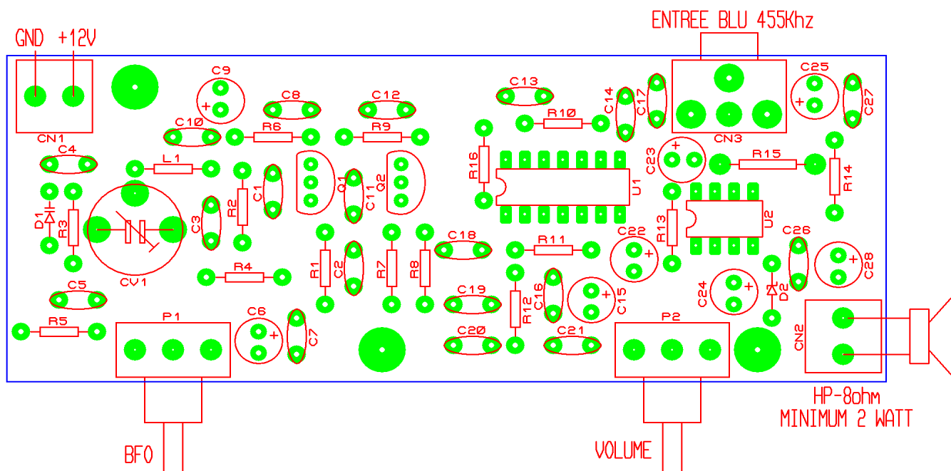
Schéma d'implantation
