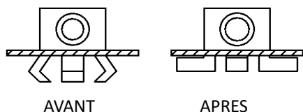
CONNECTEUR RCA
