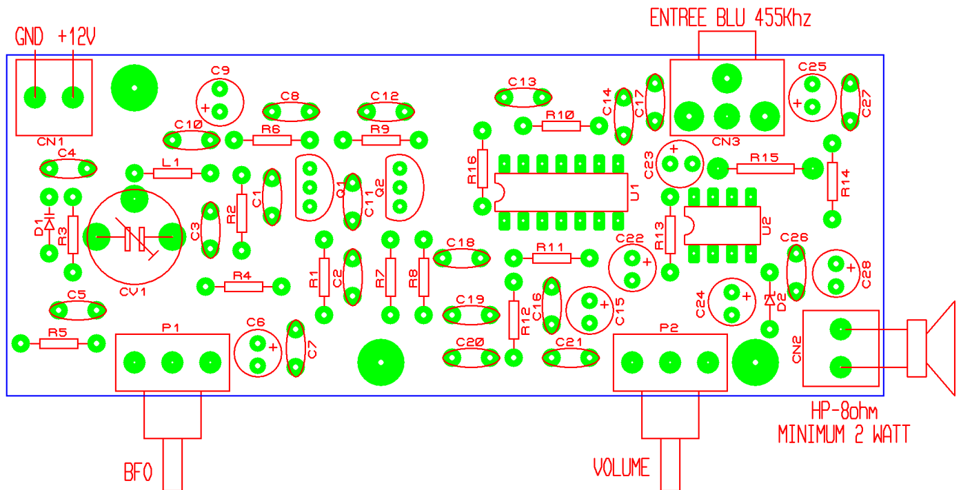
Schéma d'implantation
